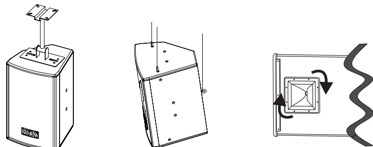
吊挂吊装
